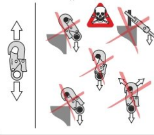
Рис. 5. Правильные и неправильные способы использования соединительных элементов
