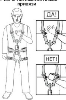
Рис. 6. Натяжение лямок привязи
