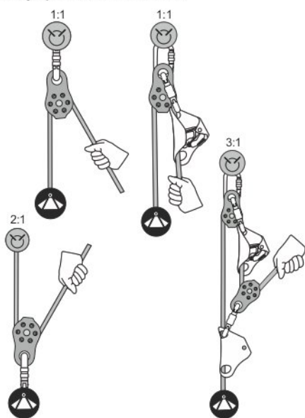
Рис. 3. Популярные схемы полиспастов
