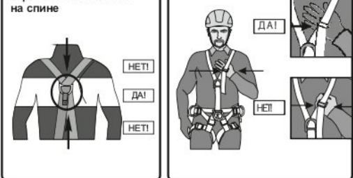
Рис. 10. Страховочная система
