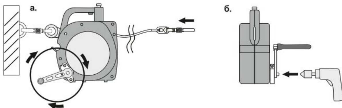
Рис. 19. Смотывание троса анкерного устройства вращением рукоятки или шуруповертом (гайковёртом)
