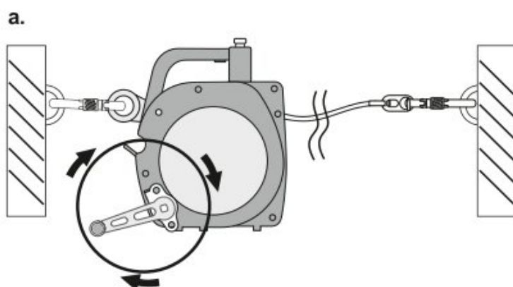
Рис. 15. Устранение провисания троса
