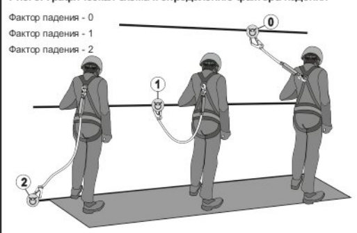
Рис. 8. Графическая схема к определению фактора падения
