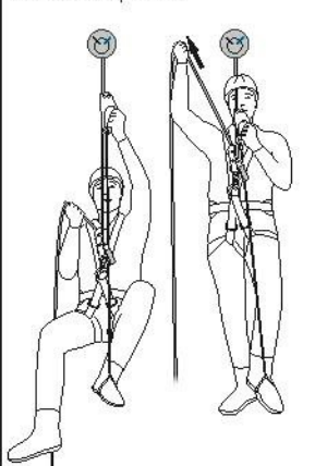
Рис. 13. Подъем с использованием зажима со стреленом
