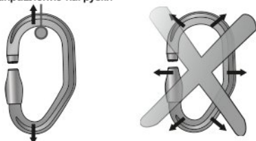
Рис. 4. Направление нагрузки
