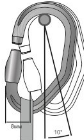
Рис. 6. Допустимый угол отклонения карабина при нагрузке
