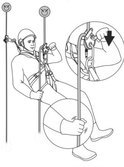
Рис. 10. Контроль каната
