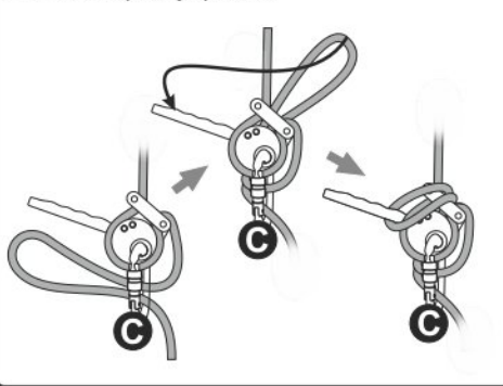
Рис. 13. Блокировка устройства
