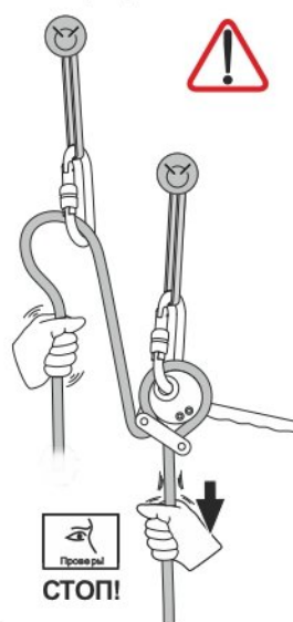
Рис. 12. Простой полиспаст
