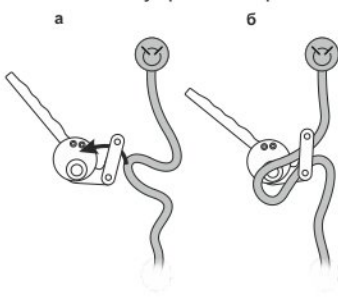
Рис. 7. Самостоятельный спуск
