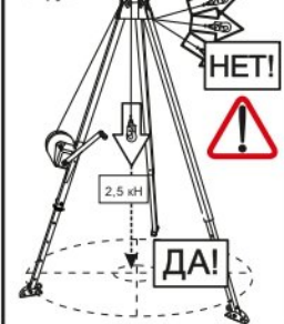
Рис. 8. Допустимое направление нагрузки
