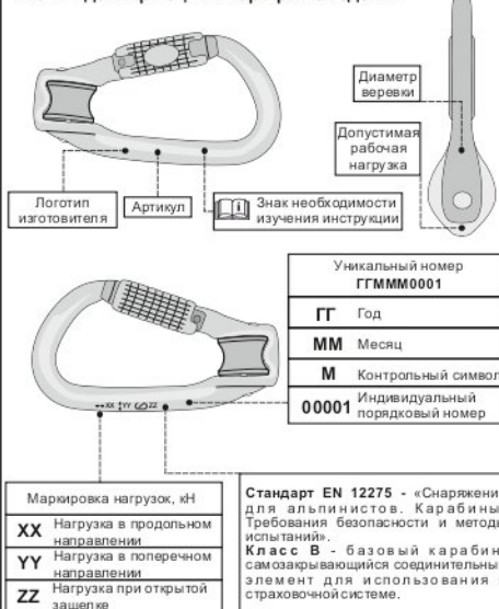
Рис. 2. Идентификация и маркировка изделия
