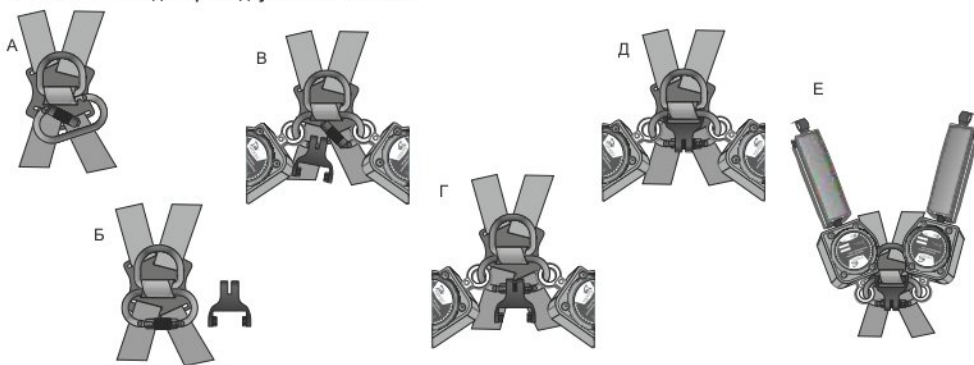
Рис. 9. Установка адаптера на двухплечевой «НВ-02»
