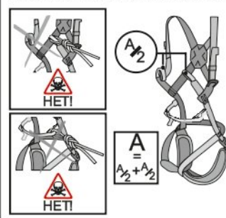
Рис. 11. Использование полных обвязок
