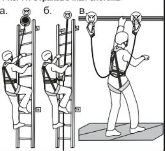
Рис. 11. Страховочная система
